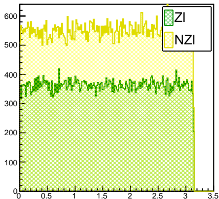
Gen Phi
