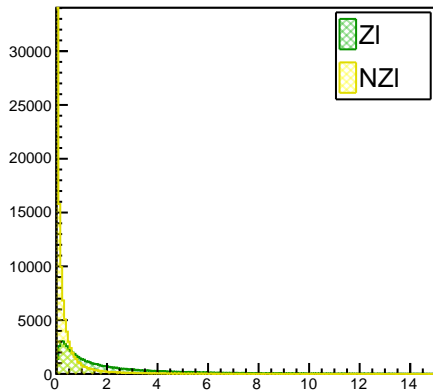
Gen Pt
