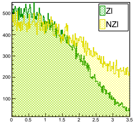
Gen Eta
