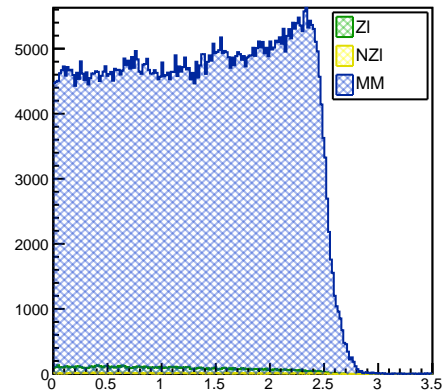
Track Eta
