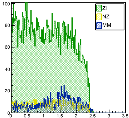
Rec Eta
