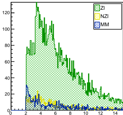
Rec Pt
