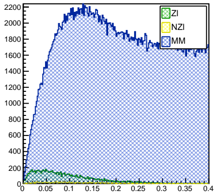
tracks_trackJetIso
