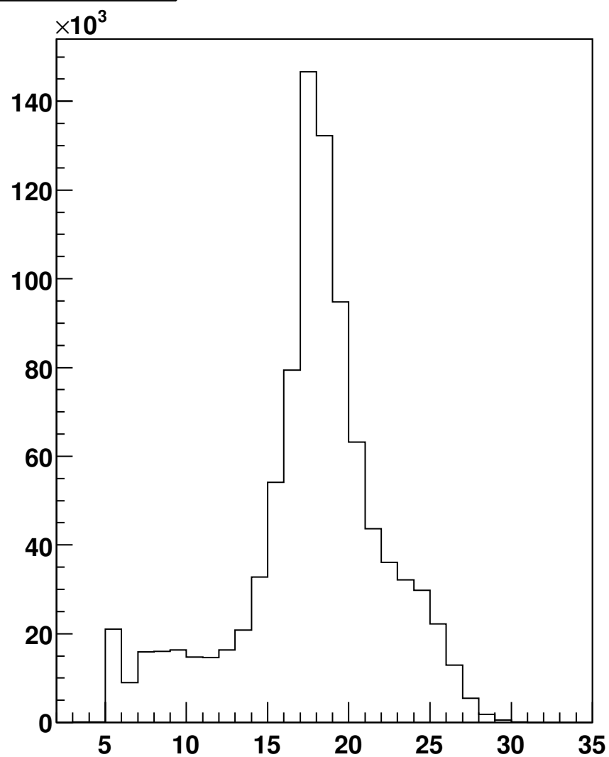
track_nHits
