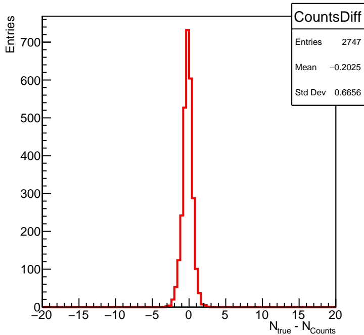
N_true - N_counts
