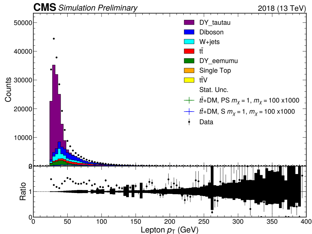
DY_jet_veto_1st_lep_pt_is_em
