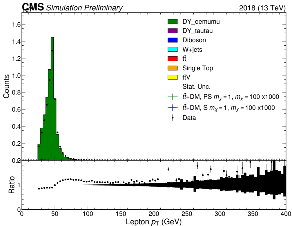
DY_jet_veto_1st_lep_pt
