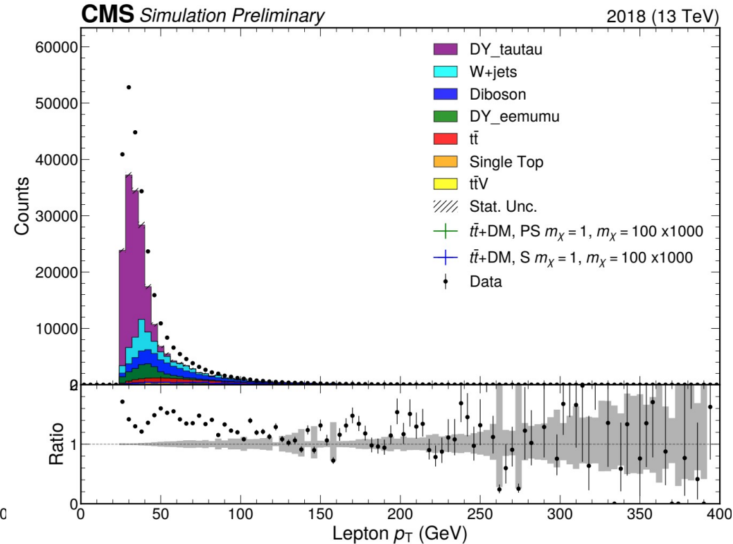
DY_jet_veto_1st_lep_pt_emu
