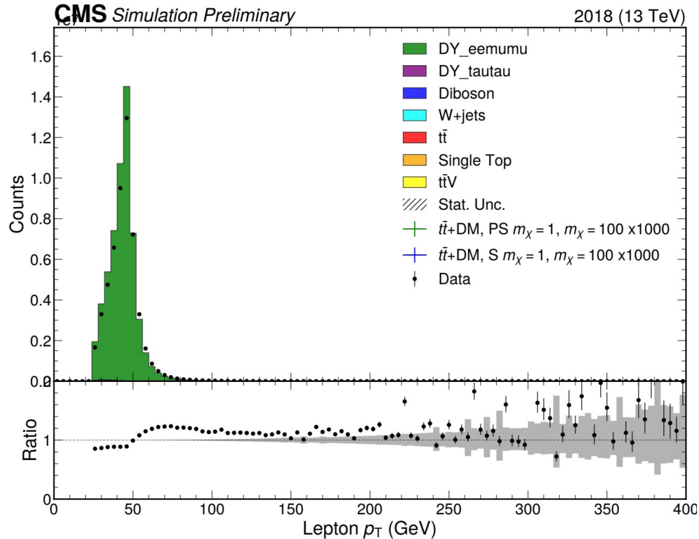
DY_jet_veto_1st_lep_pt
