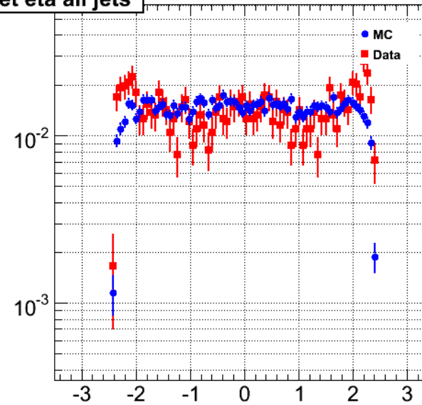
jet eta all jets
