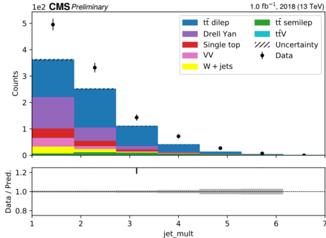
Deep CSV
