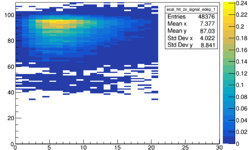
ecal_hit_zx_signal_edep_1
