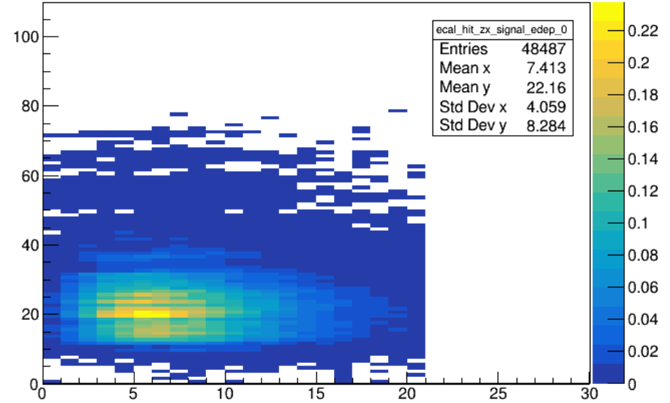
ecal_hit_zx_signal_edep_0
