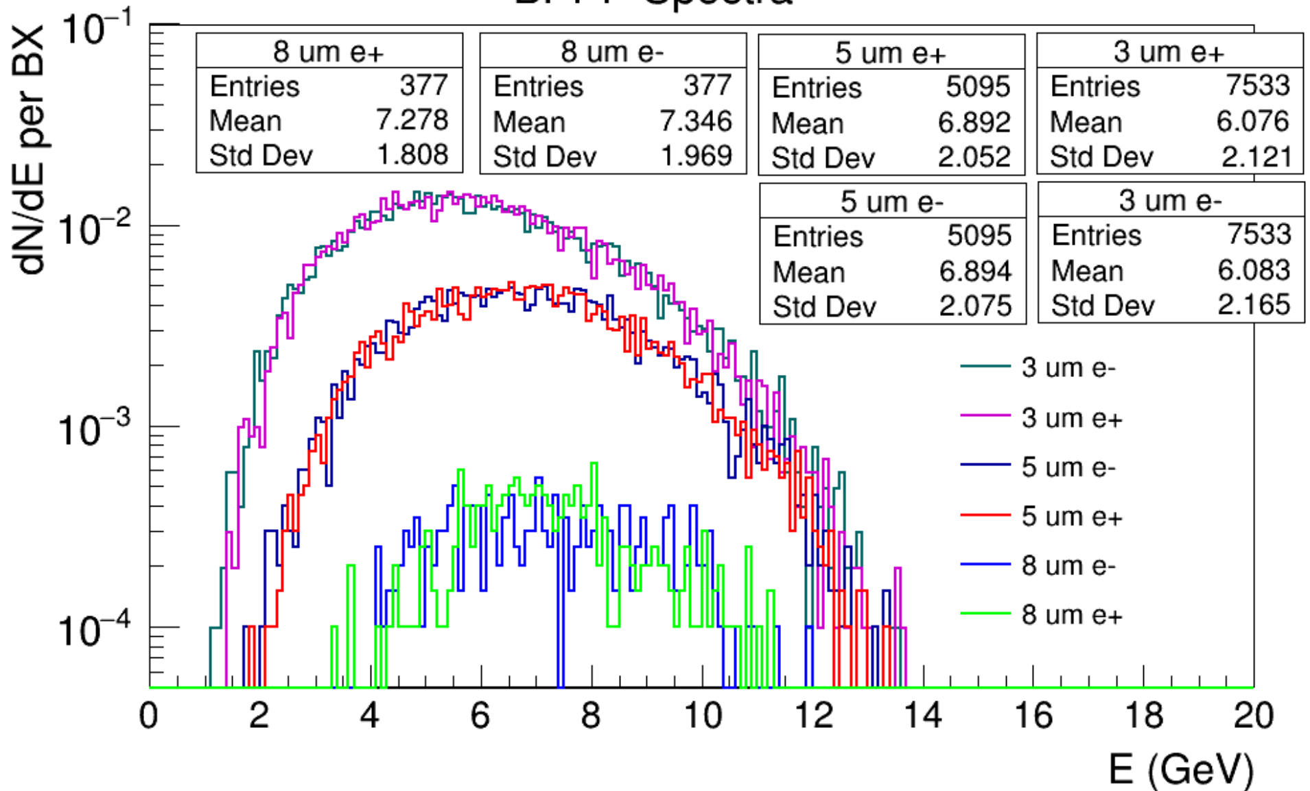
BPPP Spectra
