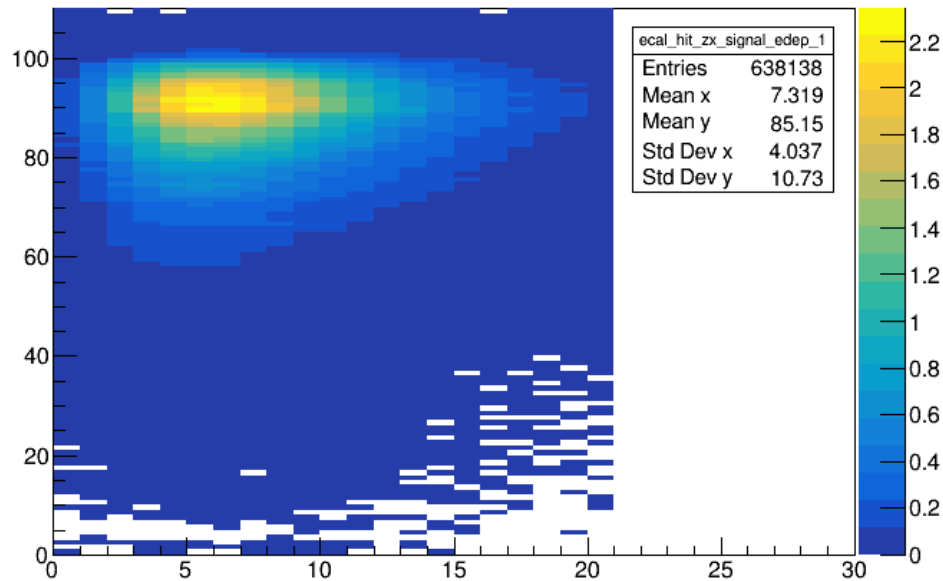
ecal_hit_zx_signal_edep_1
