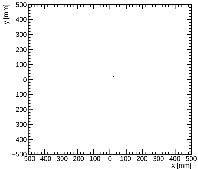
deuteron vertex y vs x for E > 0.5 GeV
