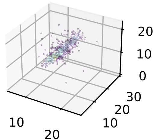
Pure Python
