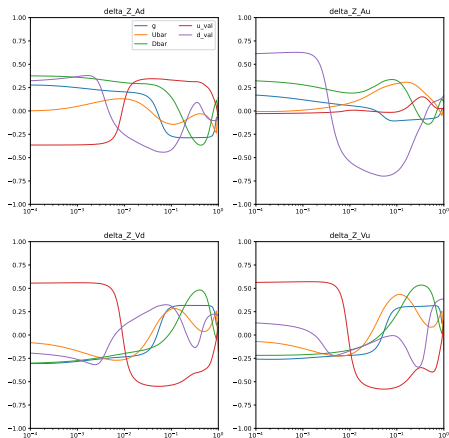
ABMP16_5_nnlo
