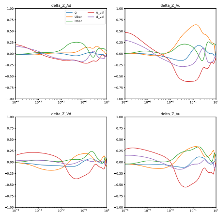
NNPDF40_nnlo_as_01180_hessian
