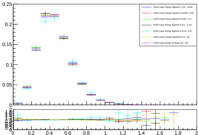
E1E2 Layer Energy - All Segments
