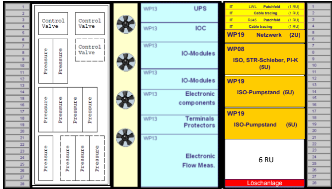
Cryo/Vakuum
