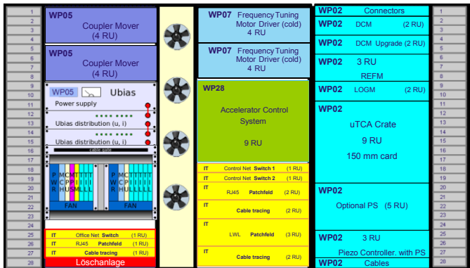
LLRF Master
