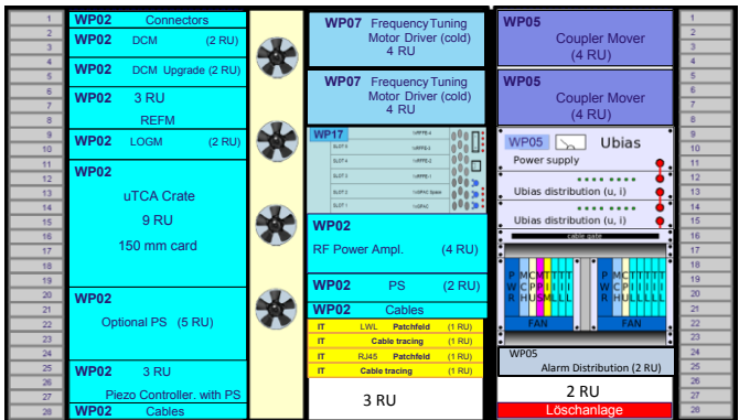
LLRF Slave
