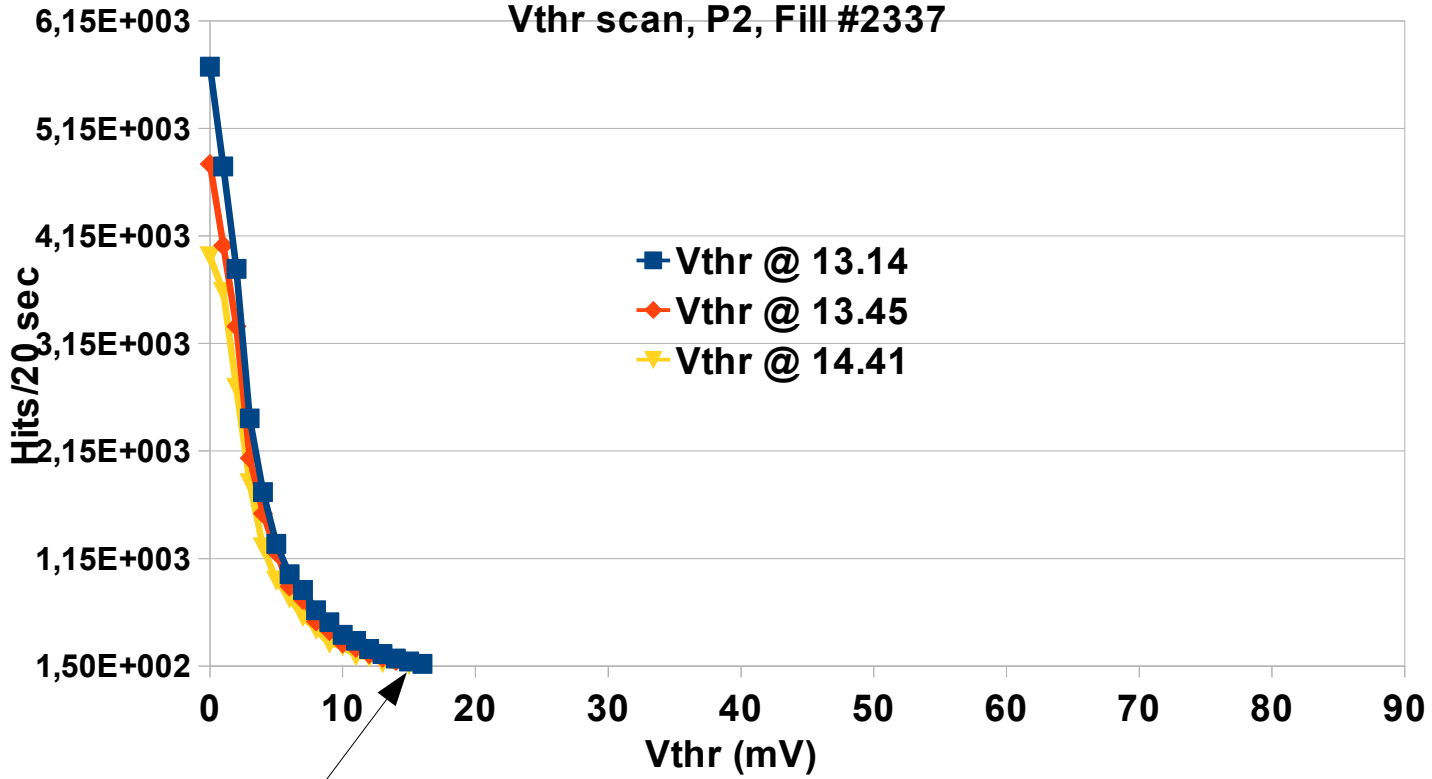
Vthr scan, P2, Fill #2337
