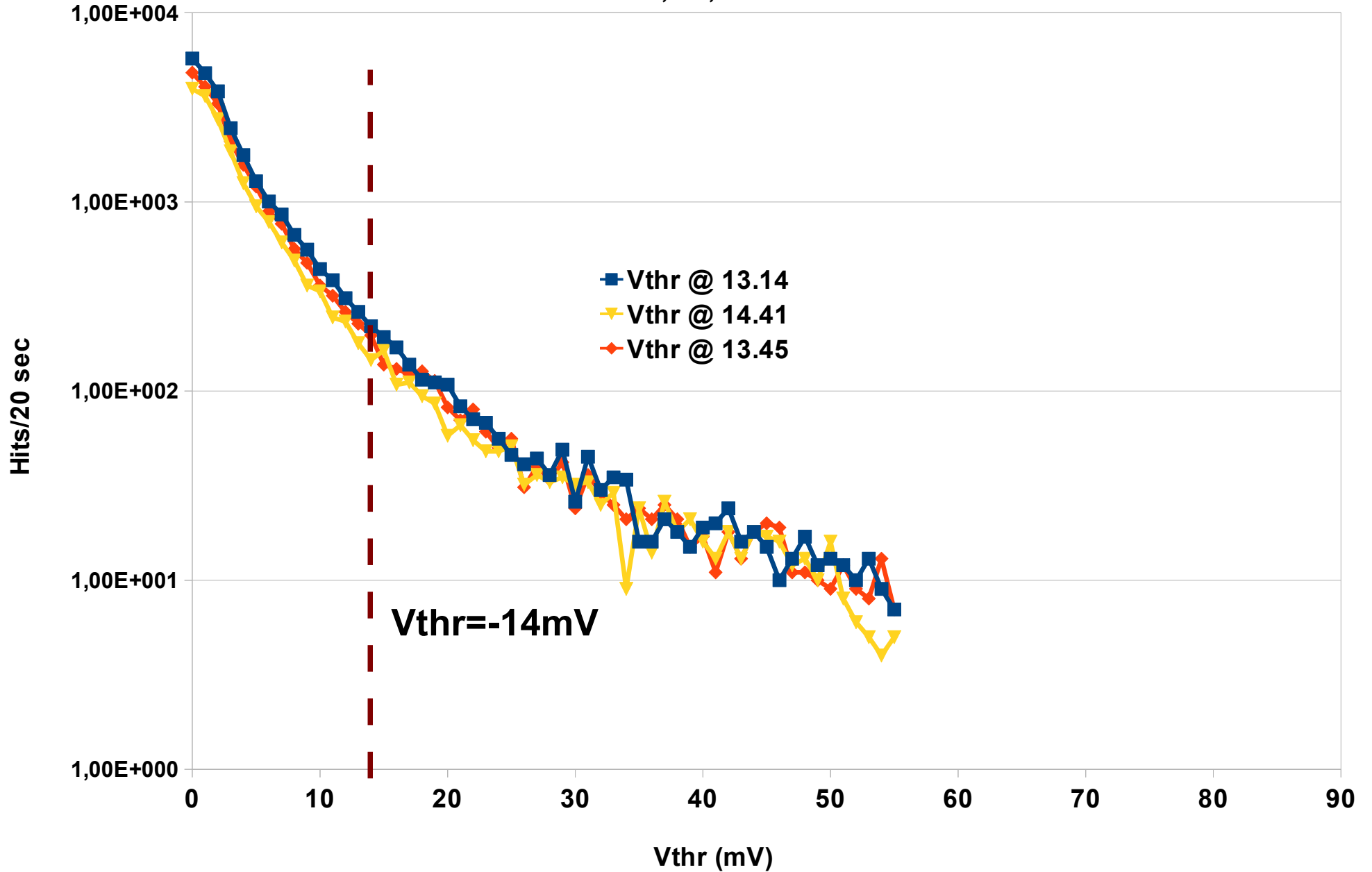
Vthr scan, P2, Fill #2337
