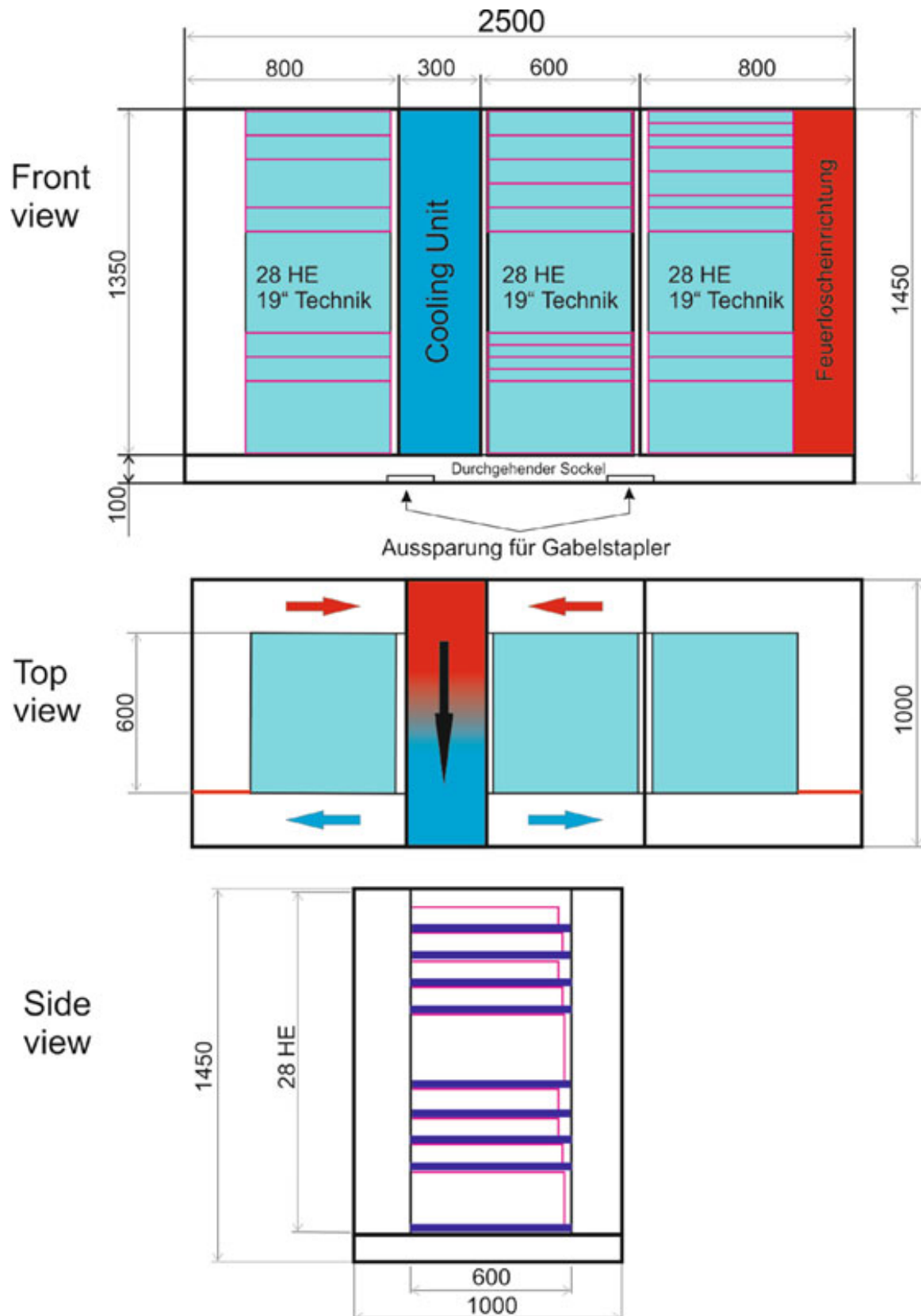
Bild 2: Beschreibung der Dreifacheinheit, Ansichten
