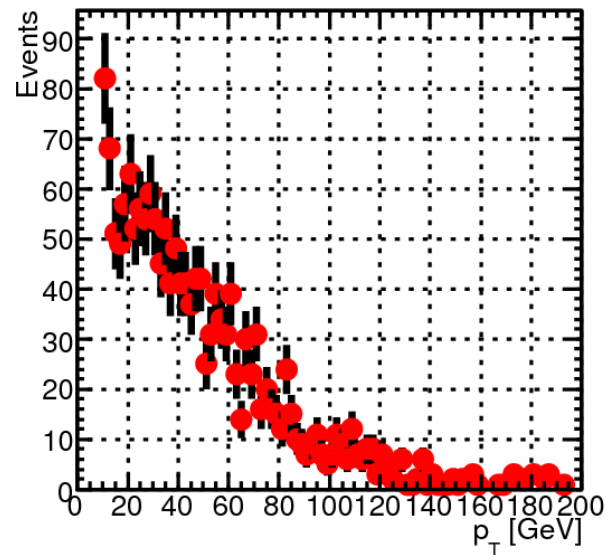
1e4j/EIPtRec
