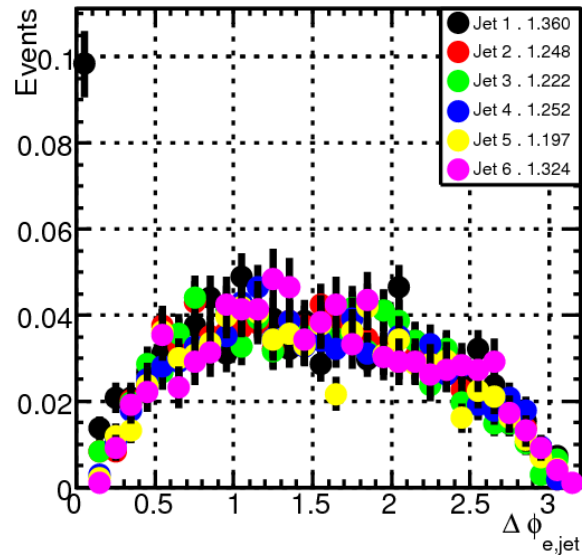
1e4j/JetDphiRec
