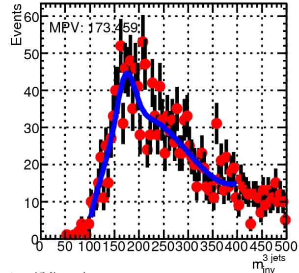
1m4j/Minv3Jet
