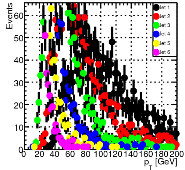
1m4j/JetPtRec
