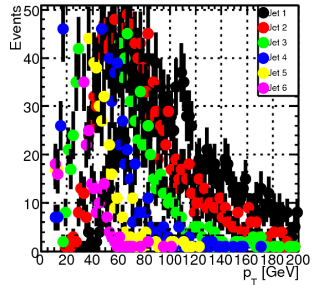
1e4j/JetPtRec
