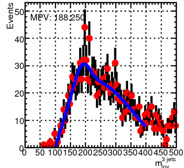
1e4j/Minv3Jet
