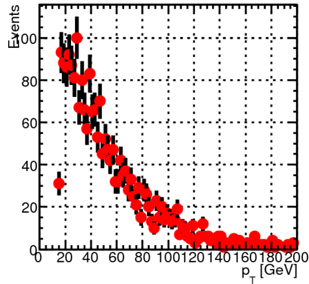
1m4j/MuPtRec
